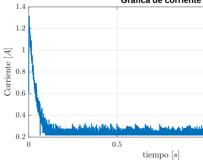
Gráfica de corriente
